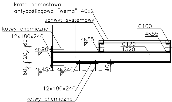
Przekrój A-A
