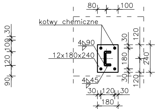
Przekrój B-B
