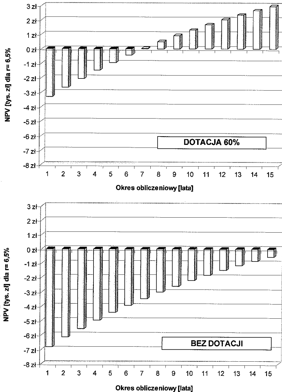
Rysunek 5.1. Strumienie środków pieniężnych w zależności od finansowania zdyskontowane w czasie żywotności inwestycji (przykład dla kotłów retortowych).
