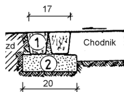
Rys. 3.3. Obramowanie wjazdu z dwóch rzędów kostki kamiennej
