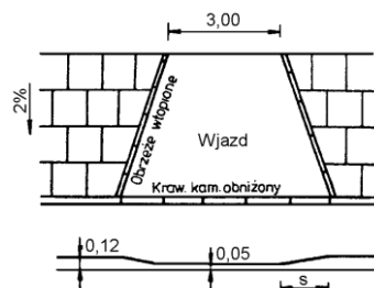
Rys. 3.2. Obrzeże wtopione jako obramowanie wjazdu
