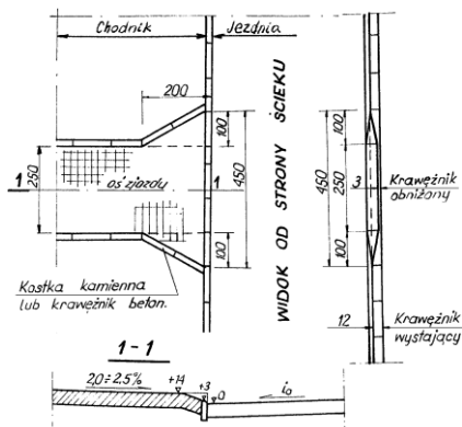
Rys. 3.1. Kształt i wymiary krawężników stosowanych jako obramowania wjazdu do bram
