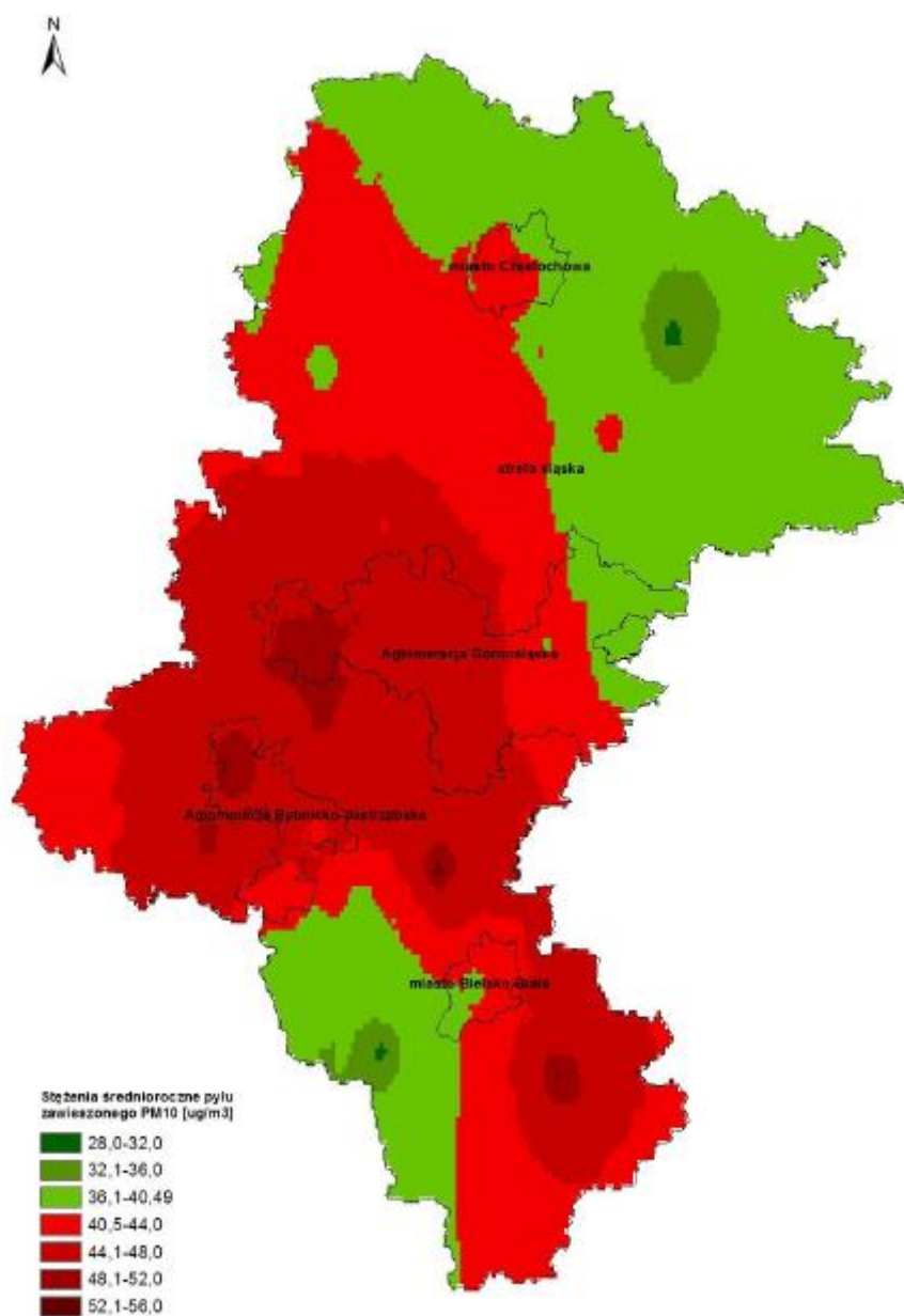
Rysunek 5-2 Obszary przekroczeń średnich stężeń rocznych pyłu zawieszonego PM10 - kryterium ochrona zdrowia ludzi
