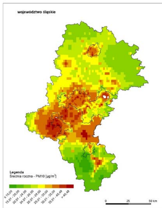
Rysunek 4. Rozkład przestrzenny średniorocznego stężenia pyłu PM10 opracowany z wykorzystaniem metody szacowania w oparciu o wyniki modelowania jakości powietrza dla 2019 roku wykonanego przez IOŚ-PIB Źródło: Roczna ocena jakości powietrza w województwie śląskim. Raport wojewódzki za rok 2019.
