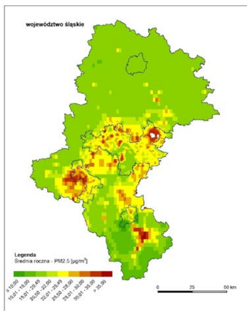
Rysunek 5. Rozkład przestrzenny średniorocznego stężenia pyłu PM2,5 opracowany z wykorzystaniem metody szacowania w oparciu o wyniki modelowania jakości powietrza dla 2019 roku wykonanego przez IOŚ-PIB Źródło: Roczna ocena jakości powietrza w województwie śląskim. Raport wojewódzki za rok 2019.
