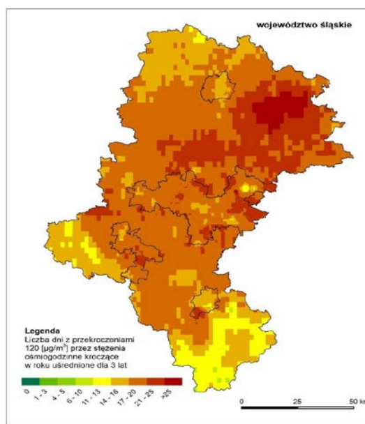
Rysunek 3. Rozkład przestrzenny liczby dni, w których najwyższa ośmiogodzinna średnia krocząca ozonu powyżej 120 µg/m 3 jest uśredniona dla trzech lat, opracowany z wykorzystaniem metody szacowania w oparciu o wyniki modelowania jakości powietrza dla roku 2019 wykonanego przez IOŚ-PIB
