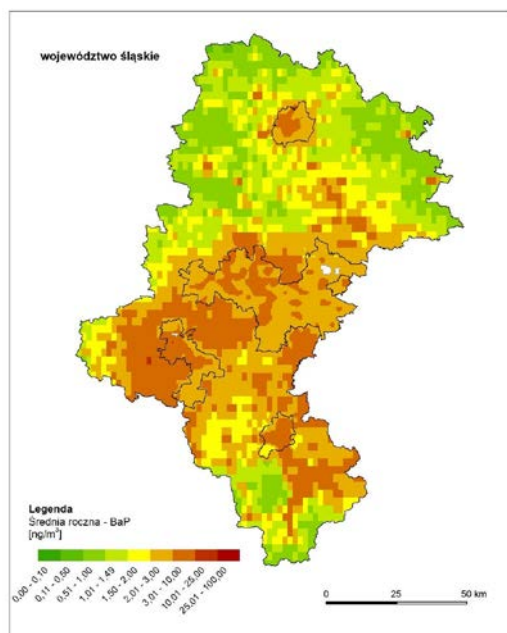
Rysunek 6. Rozkład przestrzenny stężenia średniorocznego benzo(a)pirenu opracowany z wykorzystaniem metody szacowania w oparciu o wyniki modelowania jakości powietrza dla roku 2019 wykonanego przez IOŚ-PIB
