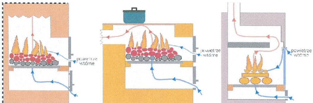
Piec kaflowy
