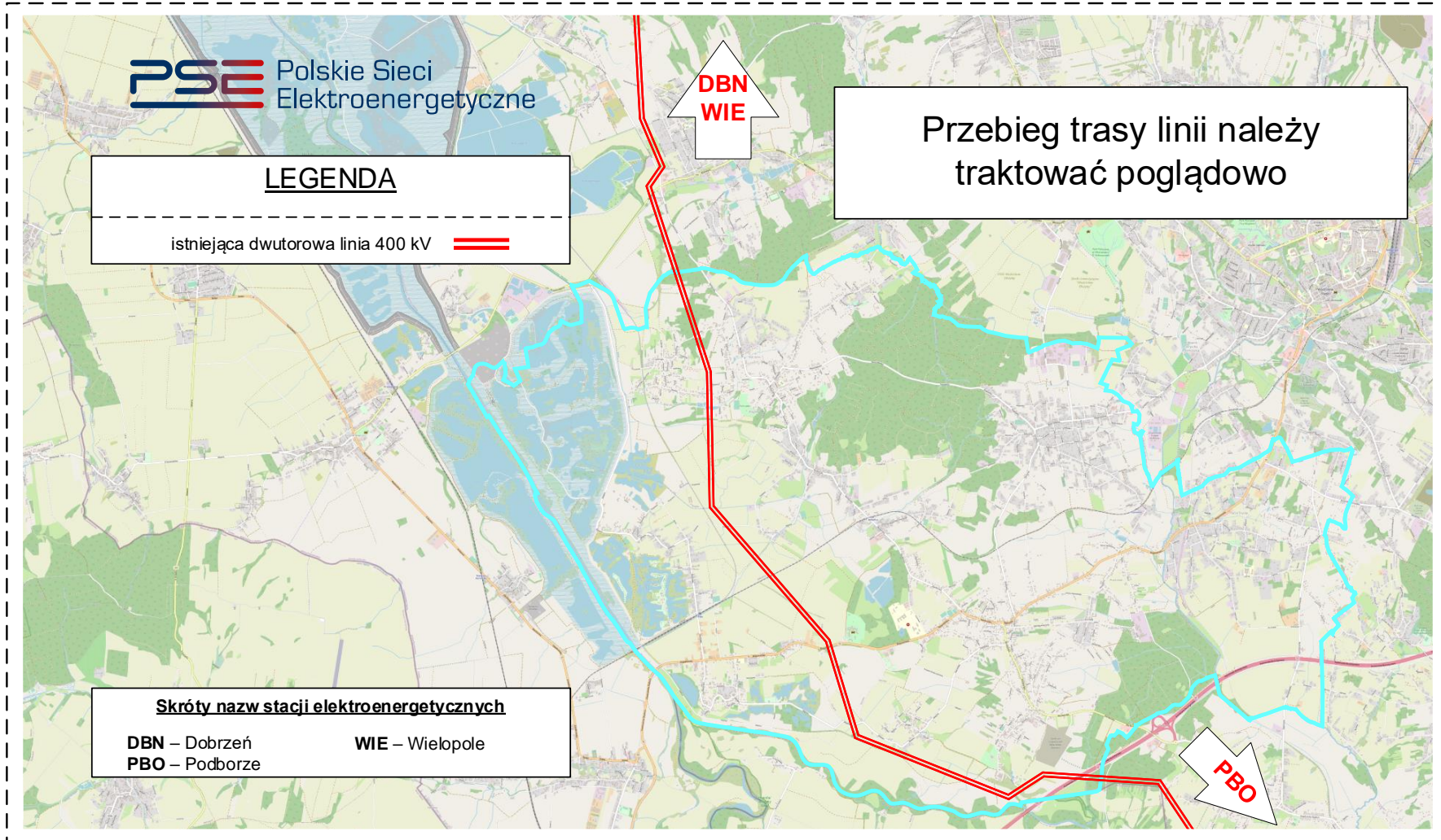
Rys. 2 Schemat sieci przesyłowej na obszarze Gminy Gorzyce – stan na 2030
